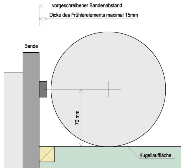
Abbildung 18 Fehlwurfanzeige
