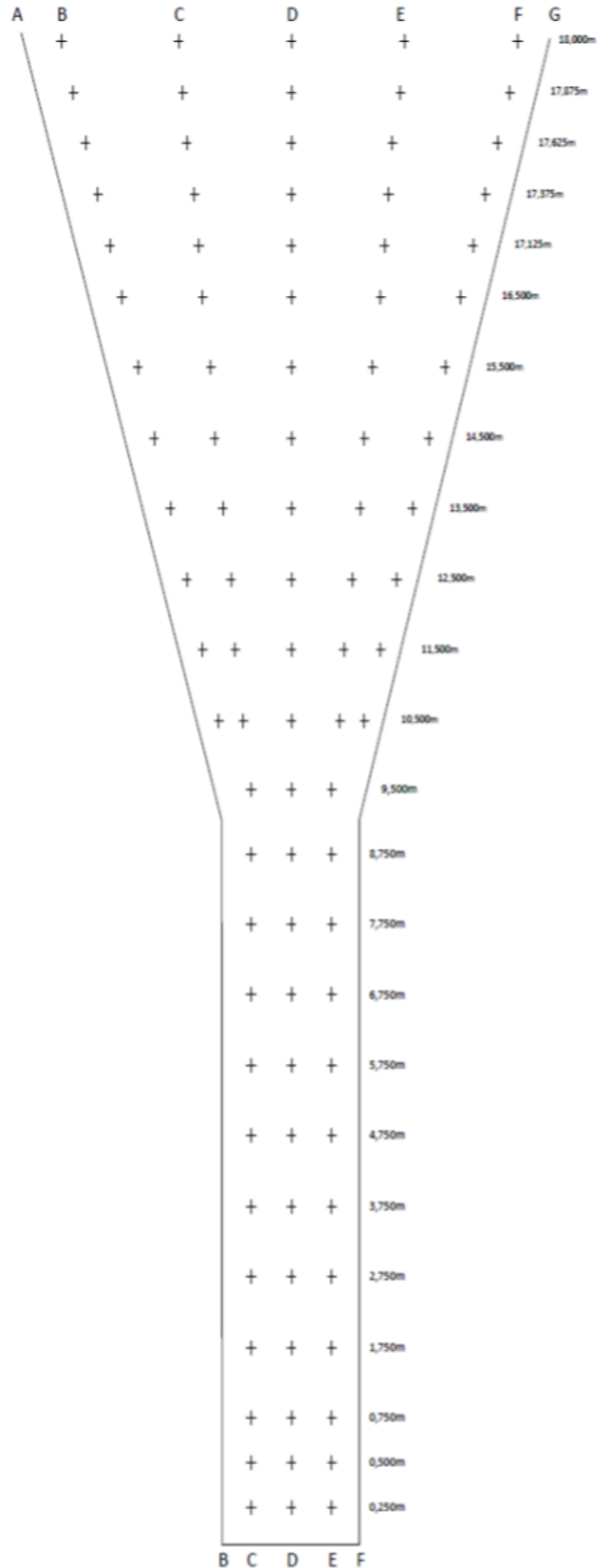
Abbildung 31: Mesststelle für Kehlung Scherenbahnen
