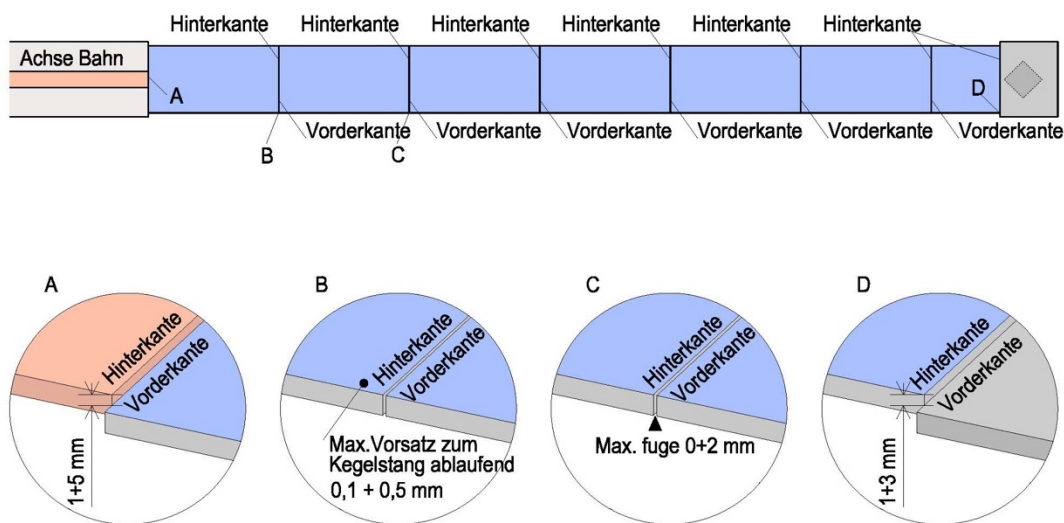
Abbildung 17 Verlegeplan Segmentbauweise
