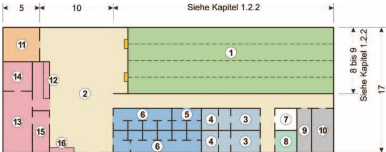
Abbildung 1 Beispiel der möglichen Anordnung der Räume einer Kegelanlage (Abmessungen in m)
